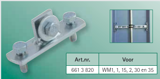
BIS Klemflens
