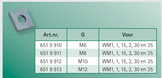
BIS Vierkantschuifmoeren
