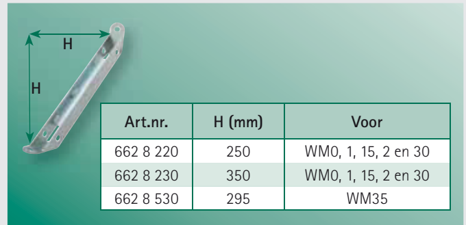
BIS Railschoren
